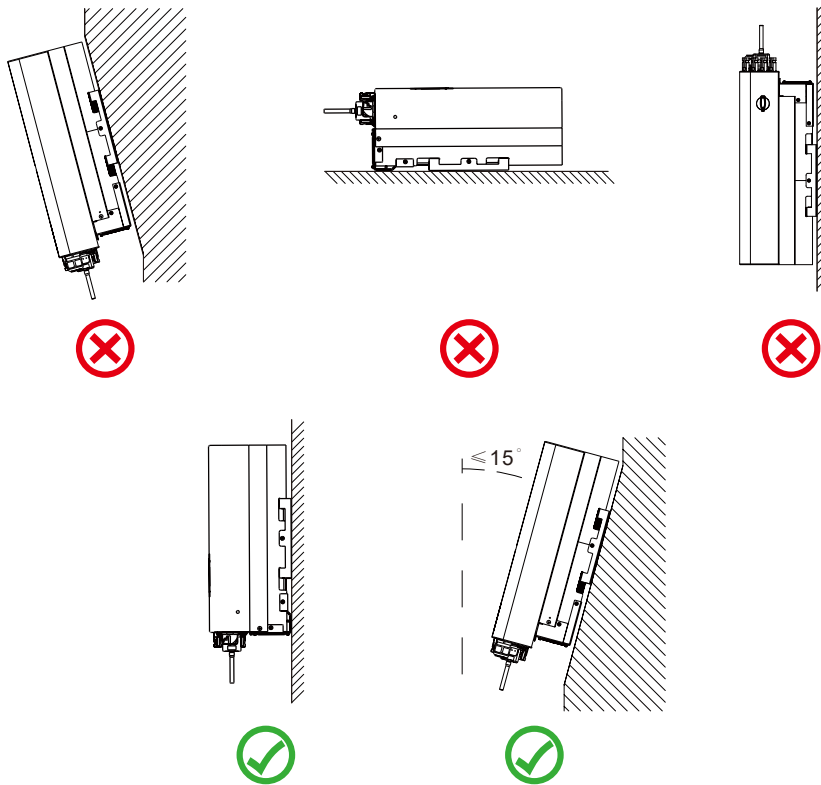
Abb. 4.2 Installationswinkel
