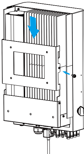
Abb. 4.6 Installation des Inverters
